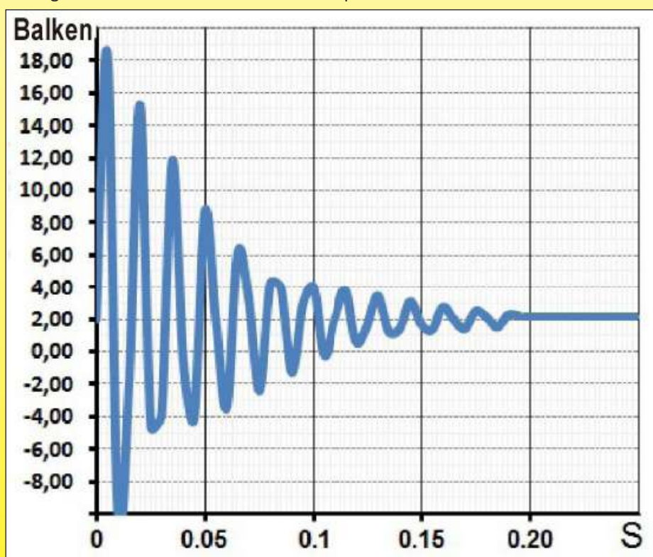
Typische Form der Druckwelle während eines Wasserschlages in einem Tank mit einem Durchmesser von 125mm, 2 bar Wasserdruck und einer Wassergeschwindigkeit von 0,5 m/s im Rohrkreislauf
